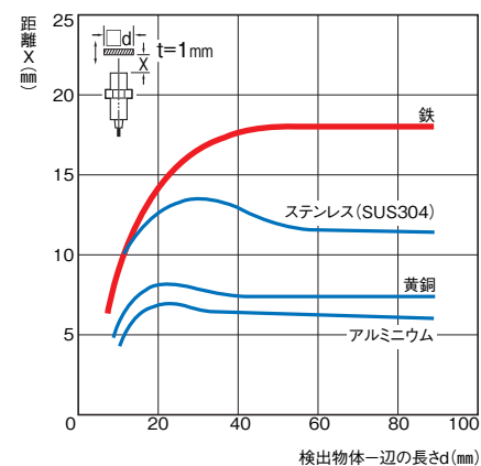
形E2E2-X18MC□/-X18MY□
