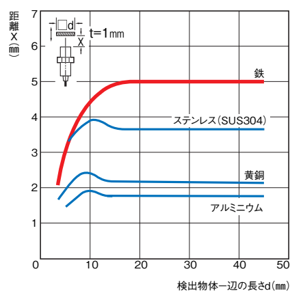
形E2E2-X10MC□/-X10MY□
