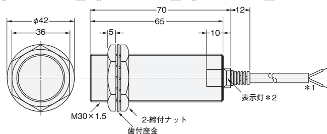
形E2E2-X10D□/形E2E2-X10C□/形E2E2-X10Y□
