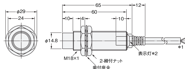
形E2E2-X14MD□/形E2E2-X10MC□/形E2E2-X10MY□
