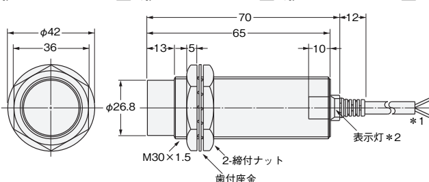
形E2E2-X20MD□/形E2E2-X18MC□/形E2E2-X18MY□
