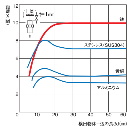
形E2E2-X18MC□/-X18MY□
