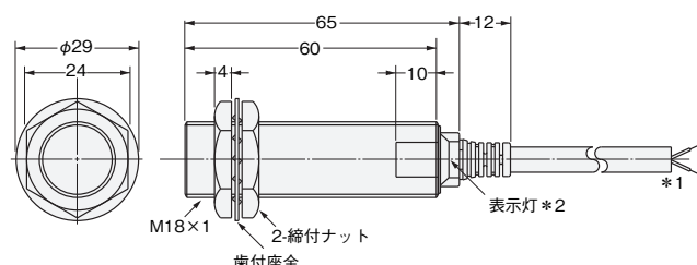
形E2E2-X7D□/形E2E2-X5C□/形E2E2-X5Y□
