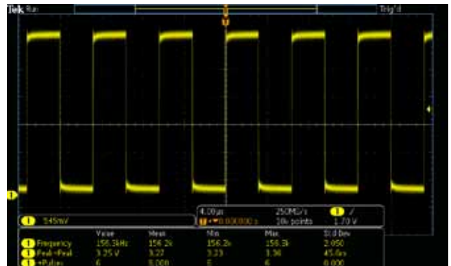
自动测量读数提供了可重复的波形特点统计视图。
