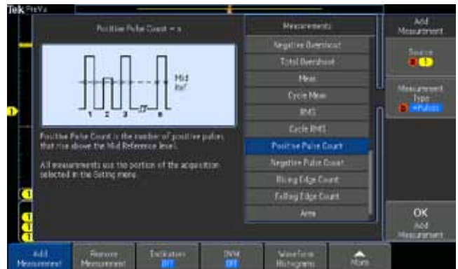
每种测量均有帮助文本以及相关图形，帮助解释如何进行测量。
