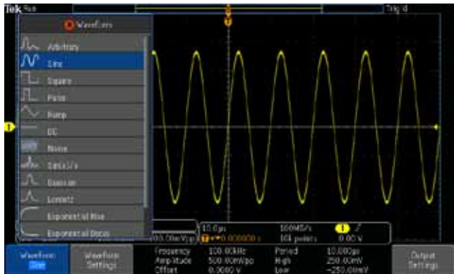
集成 AFG 中的波形类型选择
