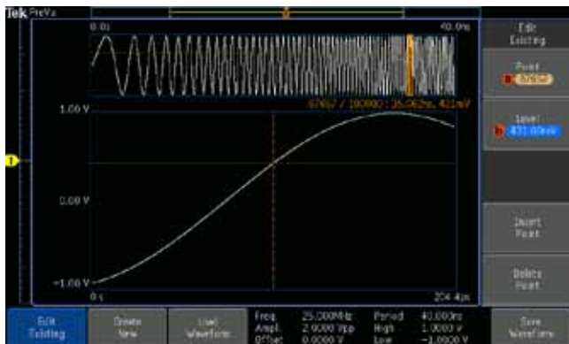
显示点到点编辑的任意波形编辑器。
