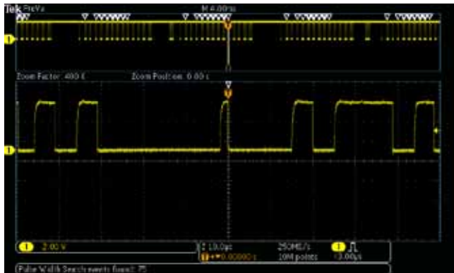
搜索步骤 2：Wave Inspector 自动搜索和记录每个事件，并用空白三角标记事件。然后可以使用 Previous 和 Next 按钮，从一个事件跳到下一个事件。
