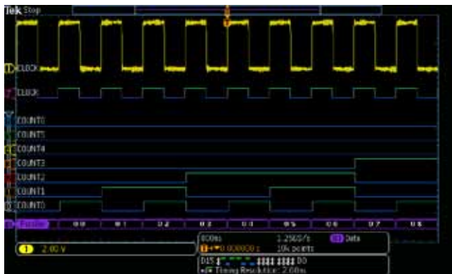
配有 MDO3MSO 的 MDO3000 系列提供了 16 条集成数字通道, 可以查看和分析时间相关的模拟和数字信号。
