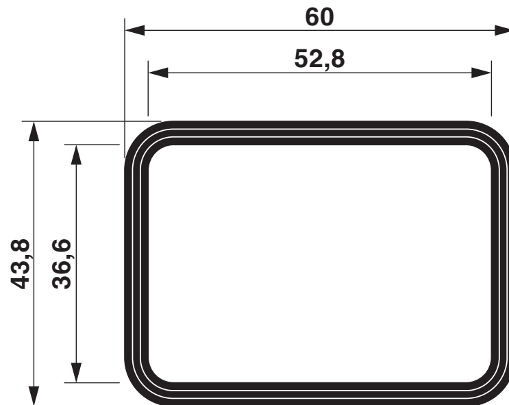
尺寸图
