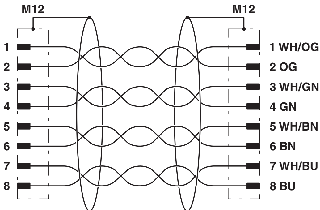
电路图
