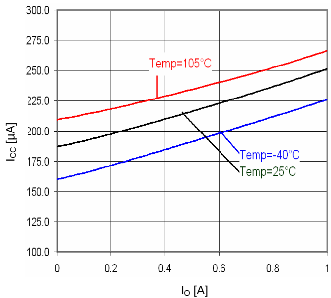
Fig.32 Io-Icc
