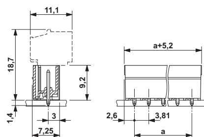
外形寸法
