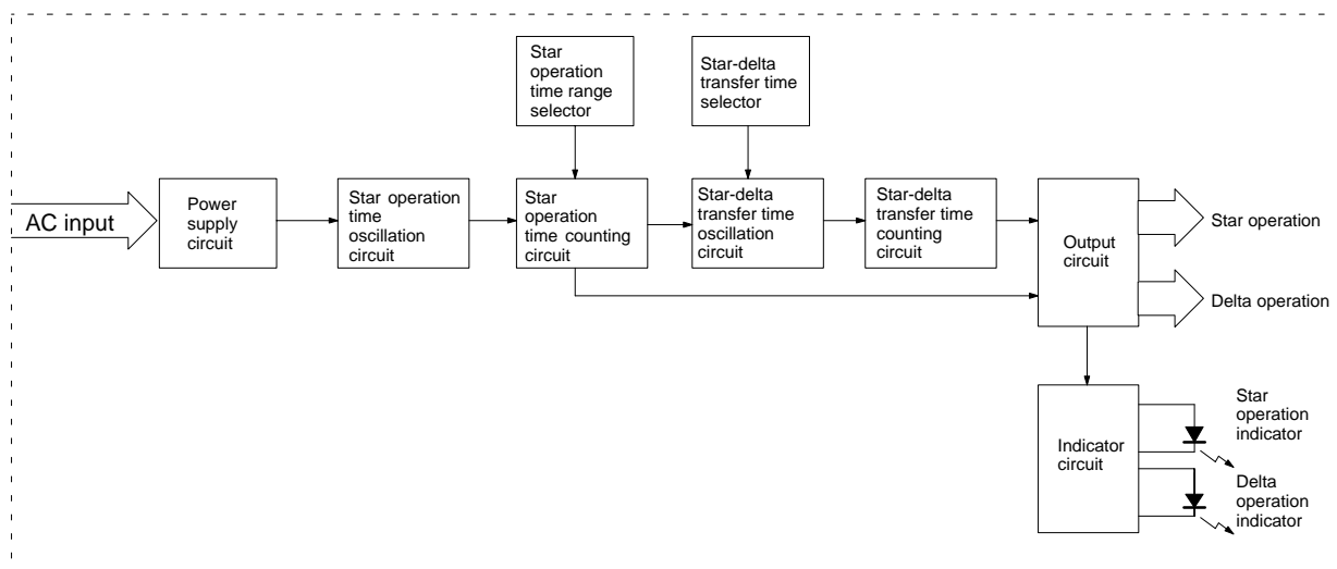
H3CR-G8L
