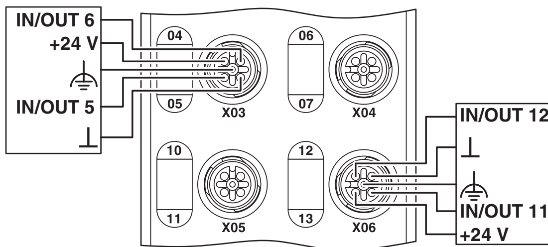
Anschlusszeichnung
