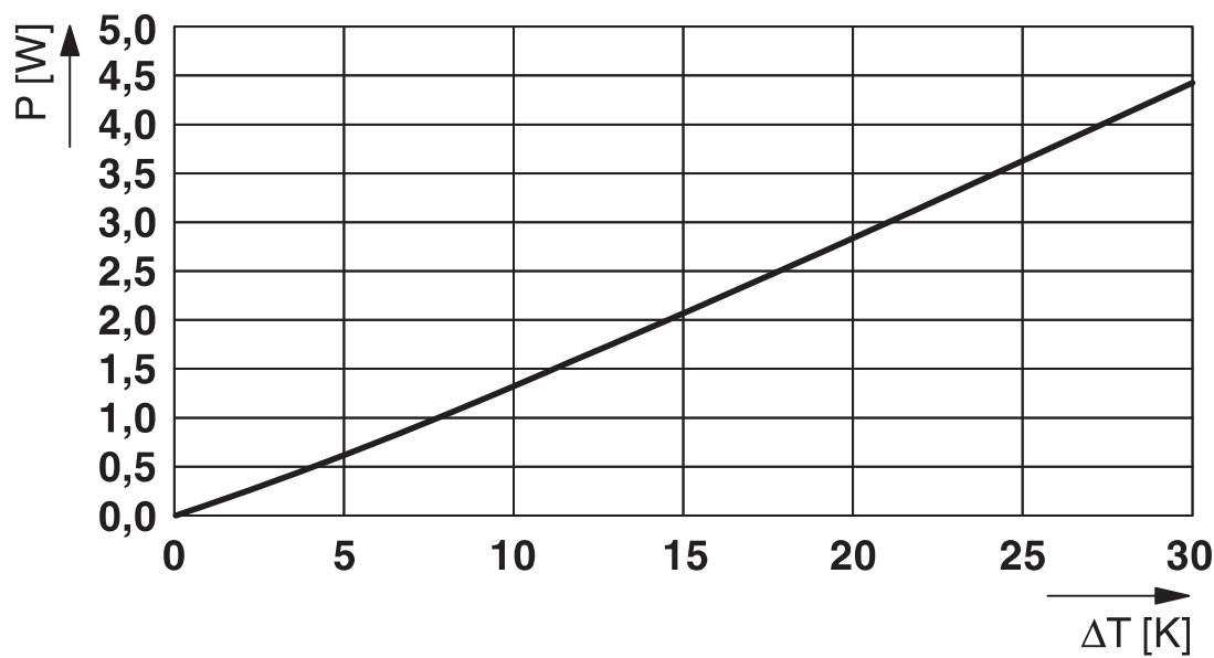
0 K ... 30 K的功耗图表
