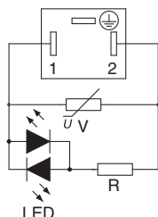
Schema del circuito DC
