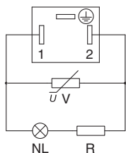
Schema del circuito AC
