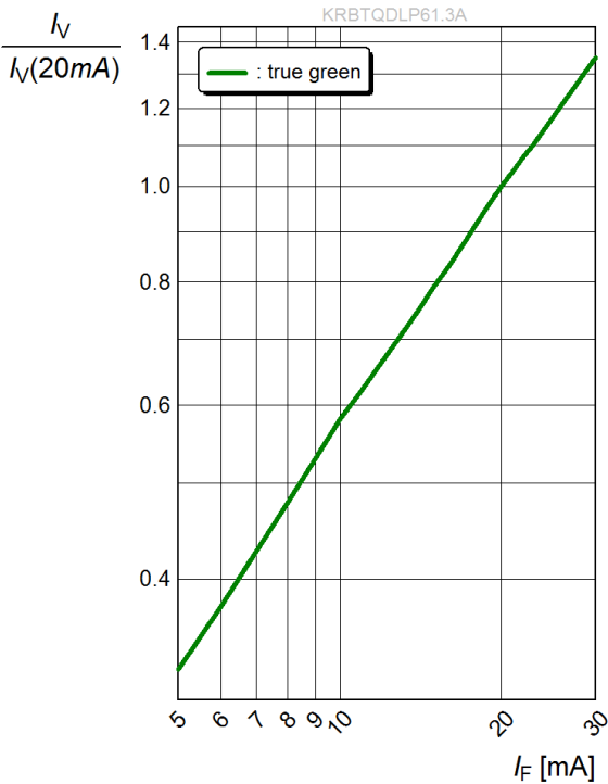
Relative Lichtstärke 8) Seite 25 Relative Luminous Intensity 8) page 25 I_V/I_V(20\text{ mA}) = f(I_F; T_S = 25\text{ }^\circ\text{C}; \text{true green})
