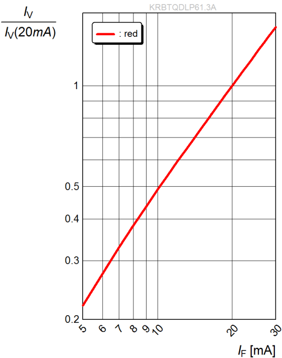
Relative Lichtstärke 8) Seite 25 Relative Luminous Intensity 8) page 25 I_V/I_V(20\text{ mA}) = f(I_F; T_S = 25\text{ }^\circ\text{C}; \text{red})
