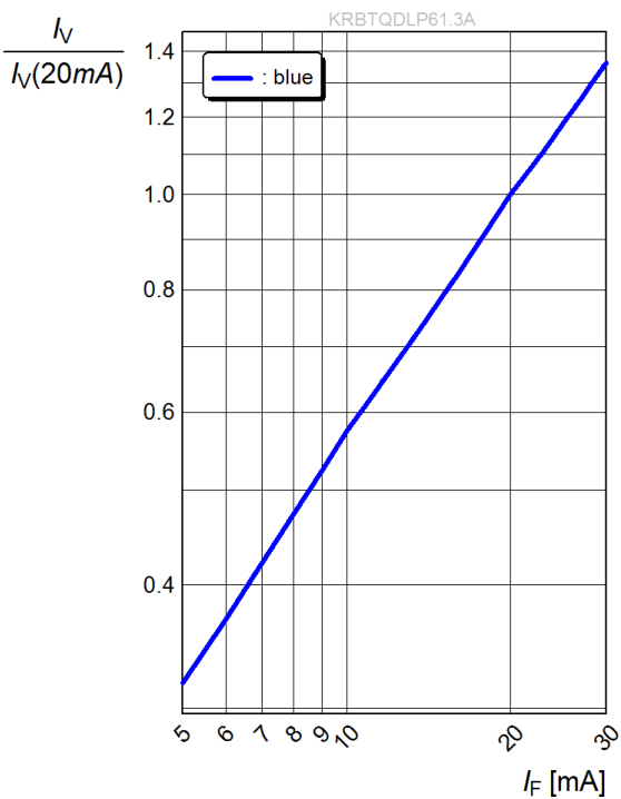
Relative Lichtstärke 8) Seite 25 Relative Luminous Intensity 8) page 25 I_V/I_V(20\text{ mA}) = f(I_F; T_S = 25\text{ }^\circ\text{C}; \text{blue})
