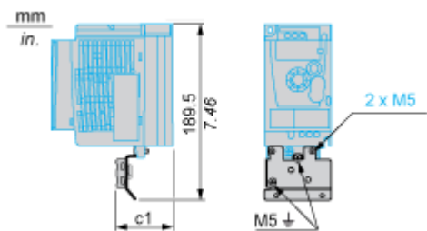
尺寸 (毫米)
