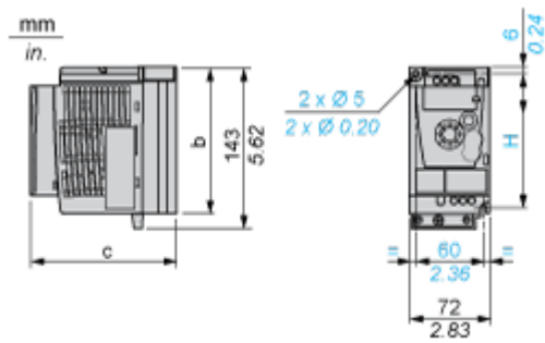
尺寸 (毫米)
