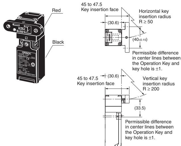
D4NS-1□F + D4DS-K3
