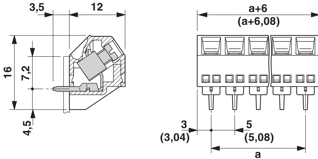
尺寸图
