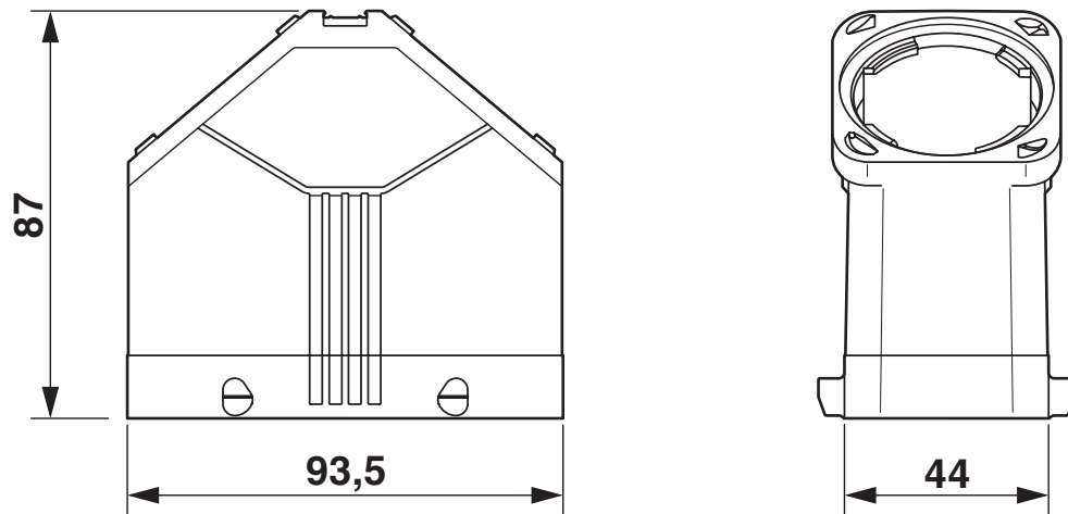
尺寸图
