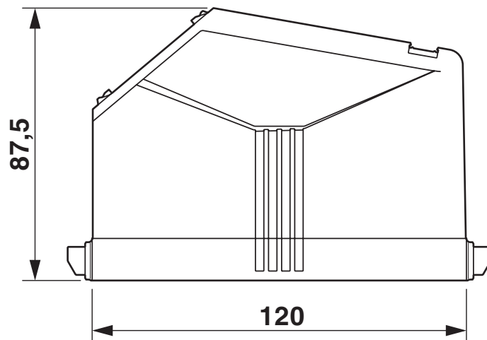
尺寸图
