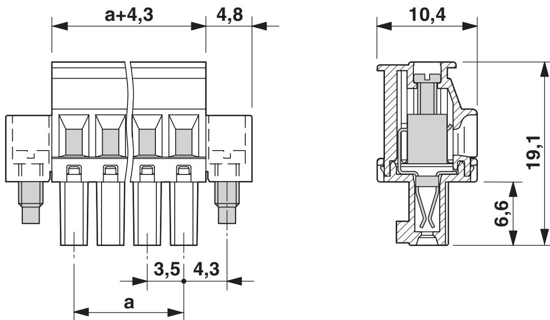
尺寸图
