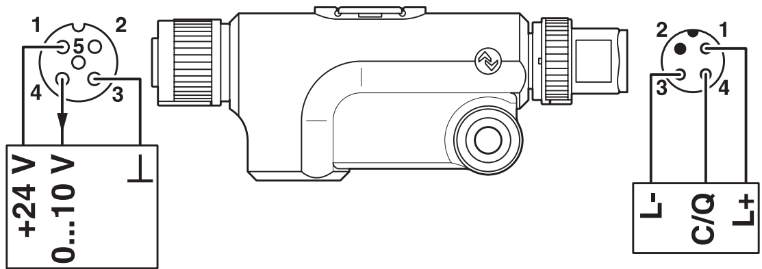
接线图
