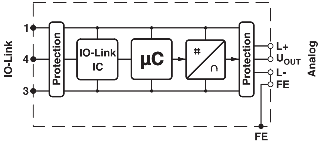
结构框图
