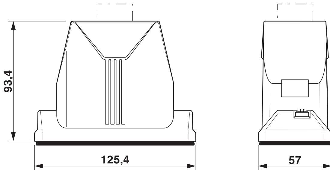
尺寸图
