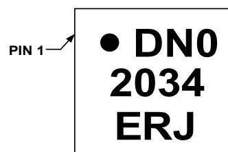
PIC18F14Q40 Example
