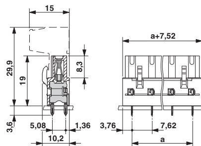
外形寸法
