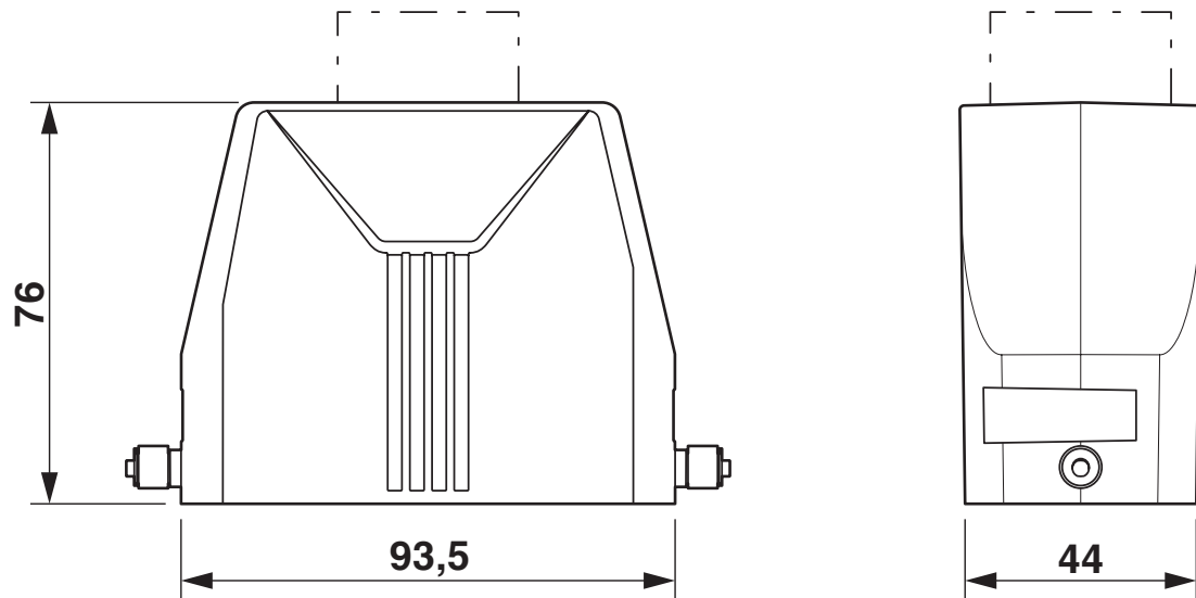
尺寸图
