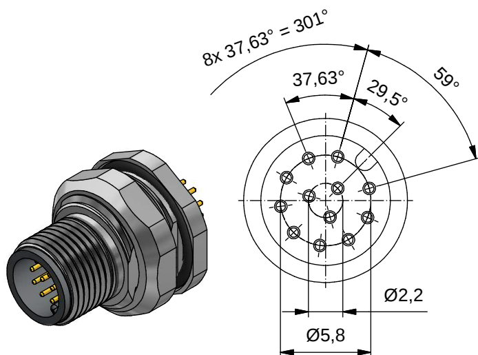
PIN layout PCB/ Lochbild Leiterplatte
