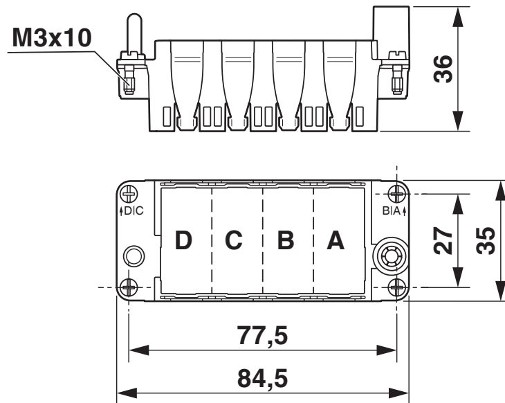
尺寸图
