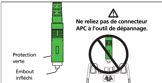
Figure 3. Identification d'un connecteur APC
