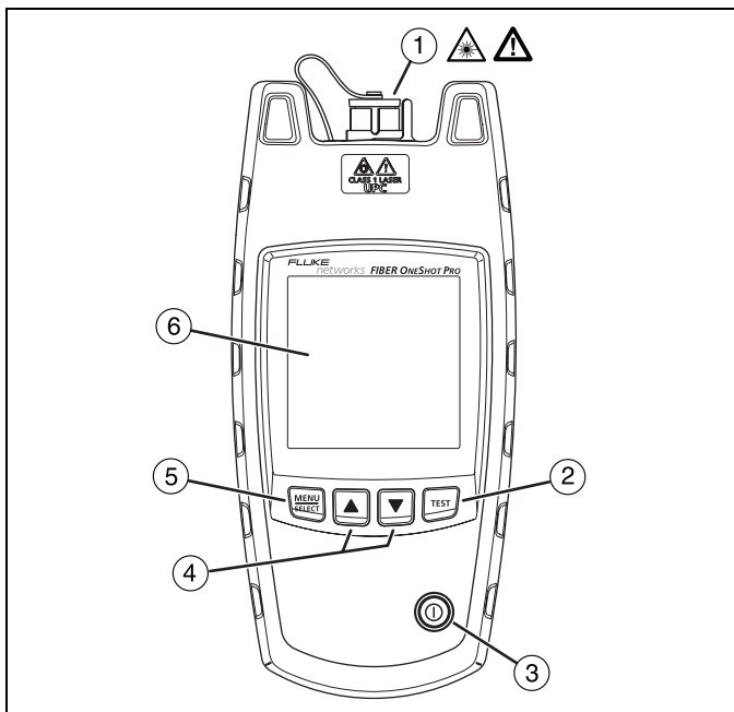
Figure 2. Caractéristiques physiques
