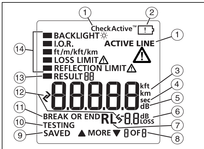
Figure 4. Fonctionnalités d'affichage
