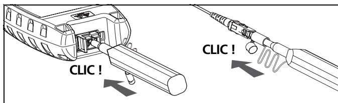
Figure 6. Nettoyage des connecteurs à l'aide d'un appareil mécanique
