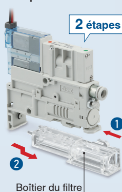
Boîtier du filtre
