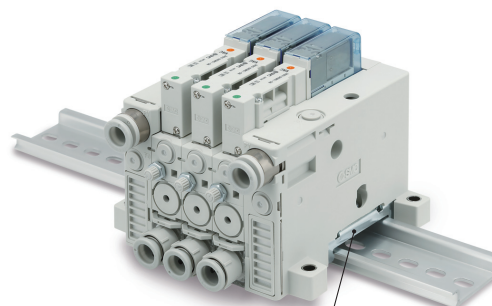
Fixation de montage sur rail DIN
