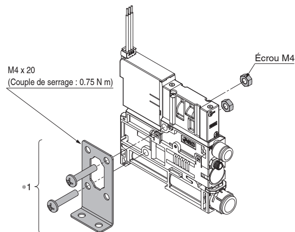
*1 Fixation pour montage individuel (option) [Écrous et vis inclus.] Référence : ZK2-BK1-A
