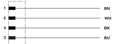
M12プラグのコンタクトアサイン
