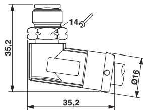
外形寸法
