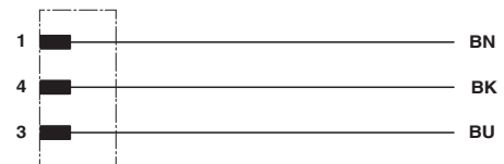
回路図
