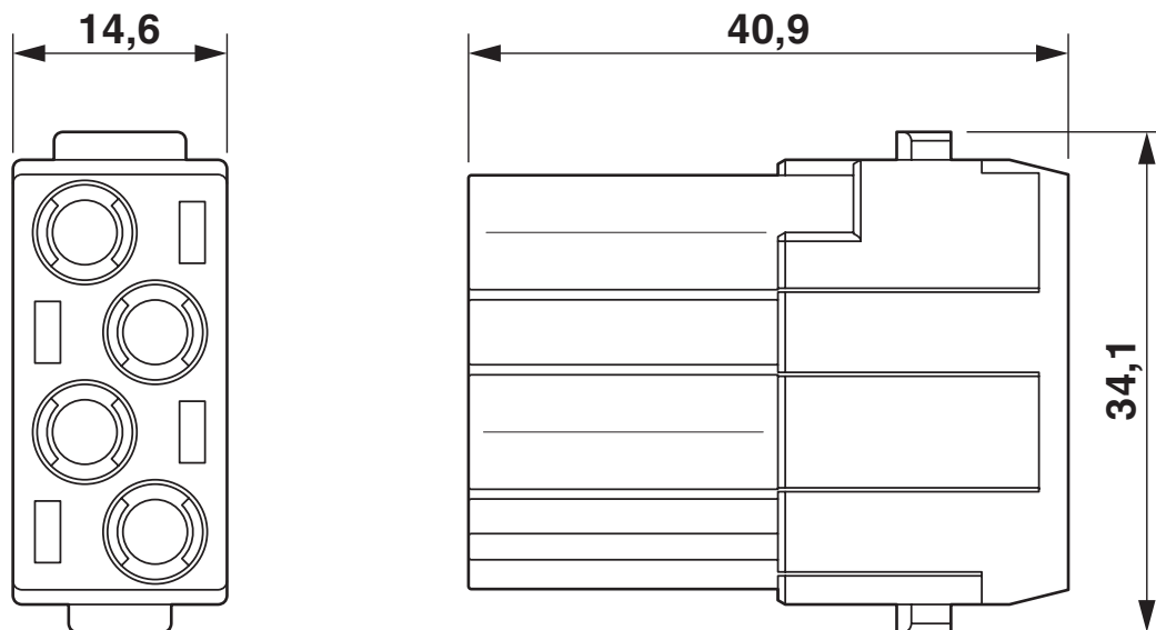
尺寸图
