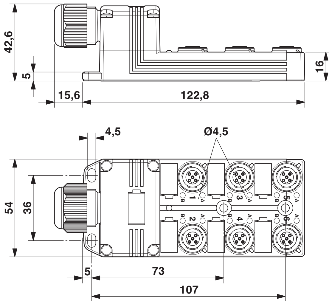
Maßzeichnung
