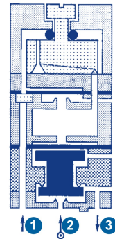
Vue du relais temporisé en 2D
