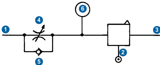
Temporisation par charge du réservoir
