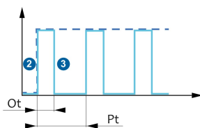
Style de courbe de temps 2
