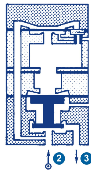
Vue du relais temporisé en 2D
