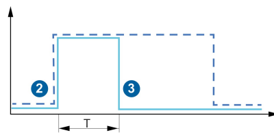
Style de courbe de temps 2 - Générateur d'impulsions unique
