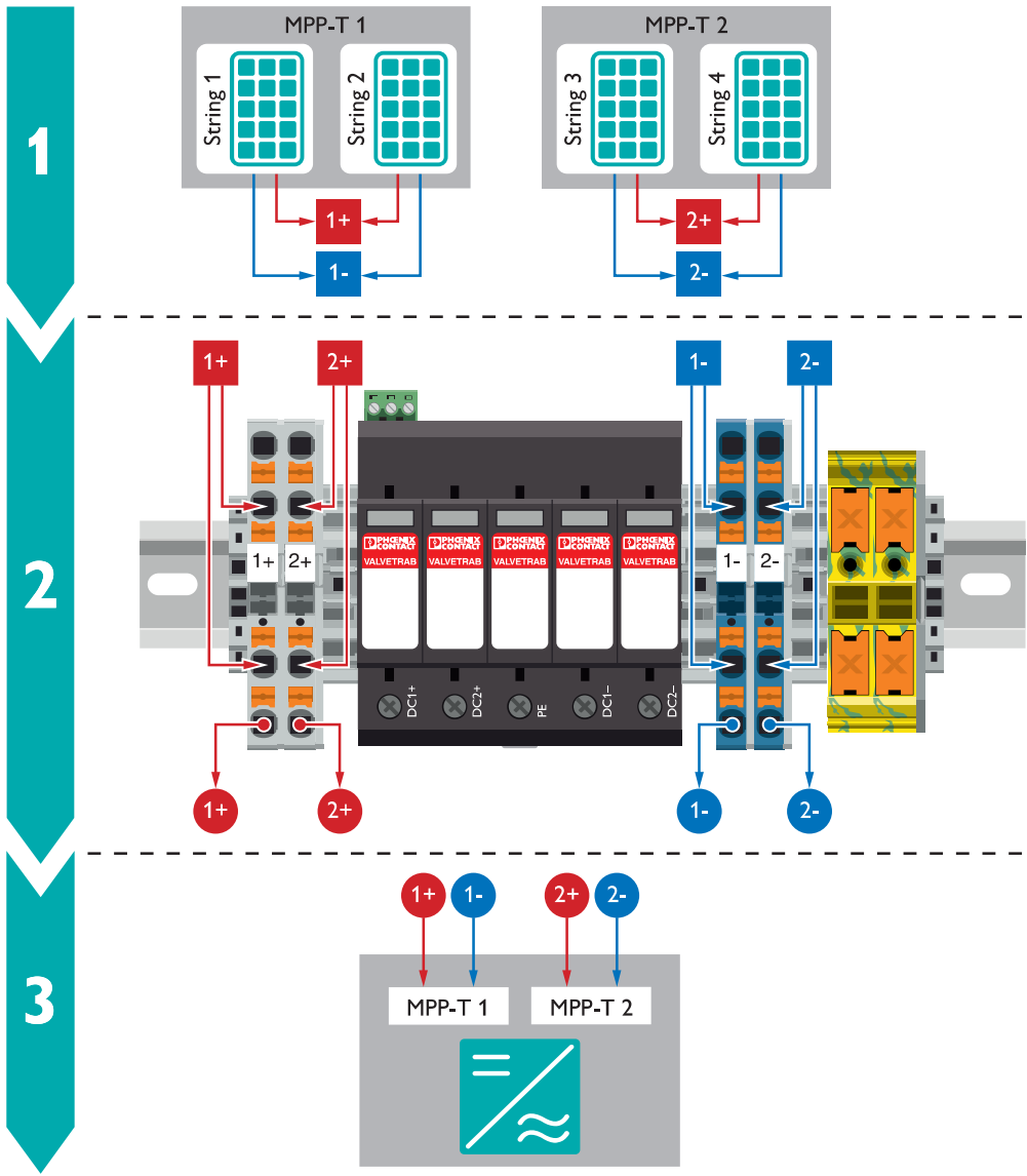
接线图
