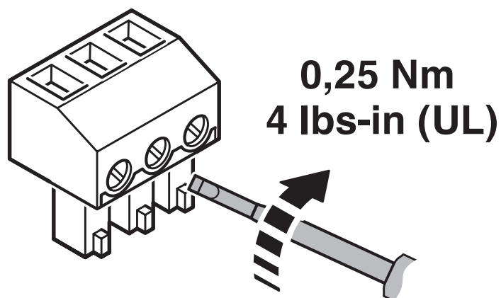
示意图
