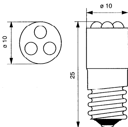
Lampensockel nach DIN EN 60061-1: E10 Lamp base in accordance to DIN EN 60061-1: E10
