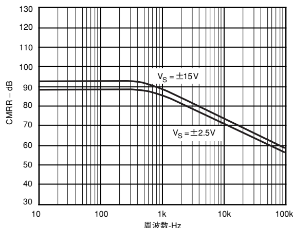
図1. AD628のCMRR対周波数特性
