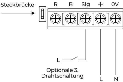
Schaltplan 2 (AC)
