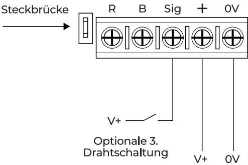
Schaltplan 1 (DC)
