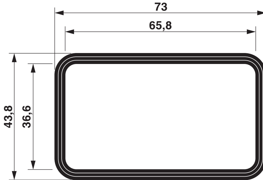
尺寸图
