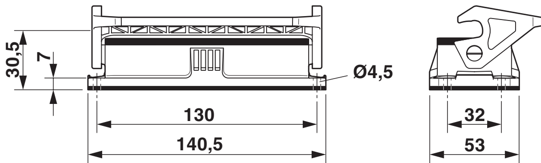
Maßzeichnung
