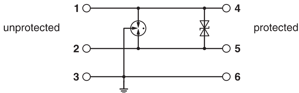
电路图
