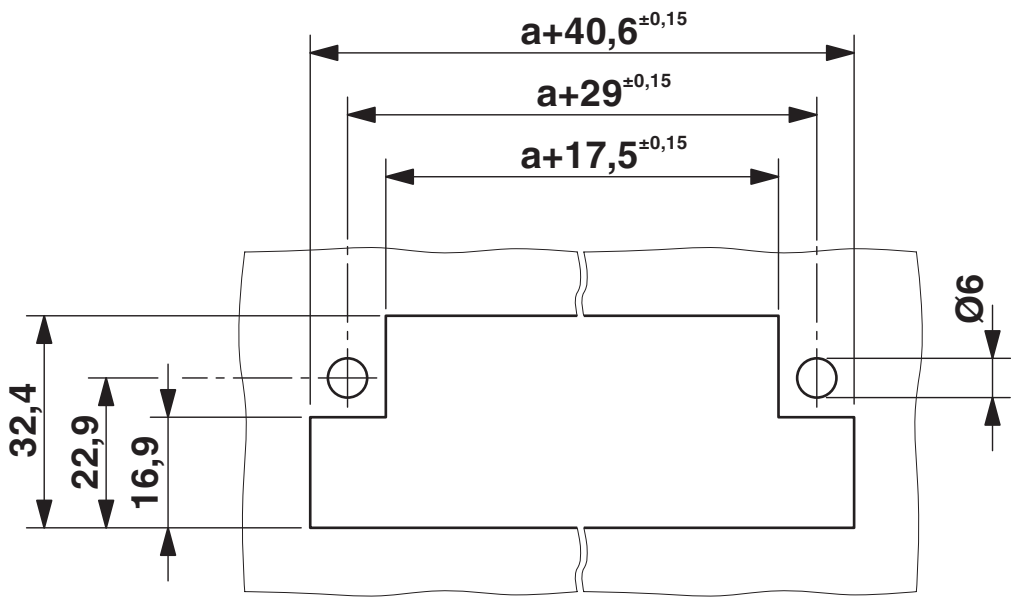
尺寸图
