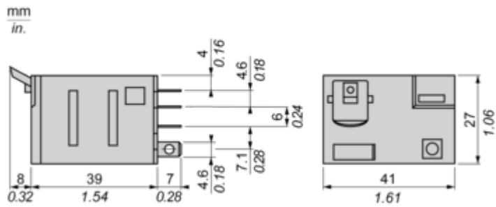
Vue côté broches
