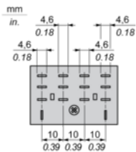
Vue côté broches
