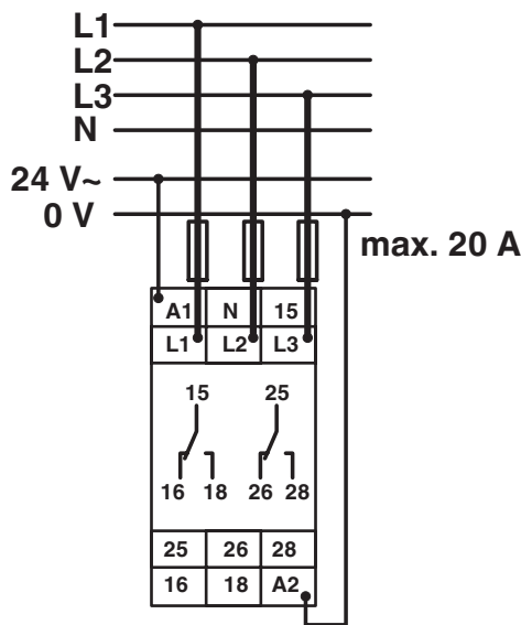
接线图
