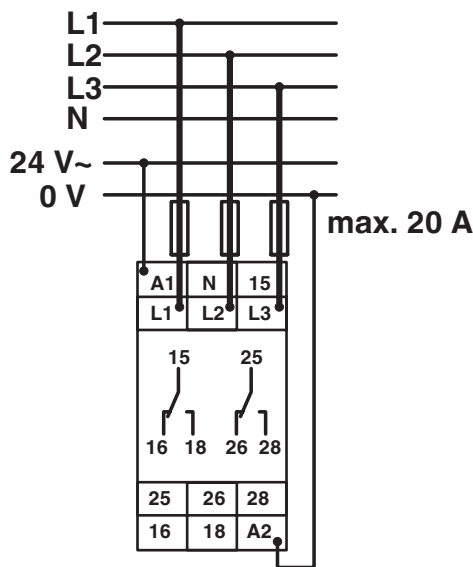
应用图
