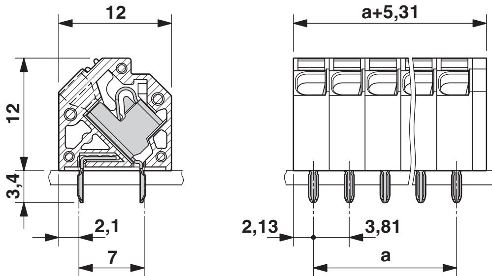
尺寸图
