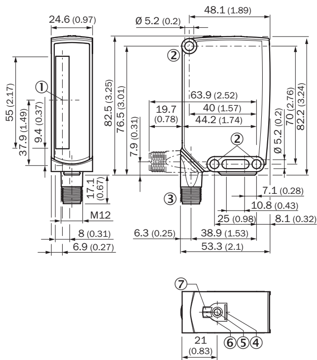
Desenho dimensional (Dimensões em mm)
