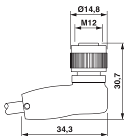
外形寸法
