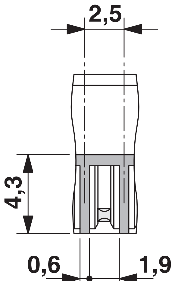
尺寸图
