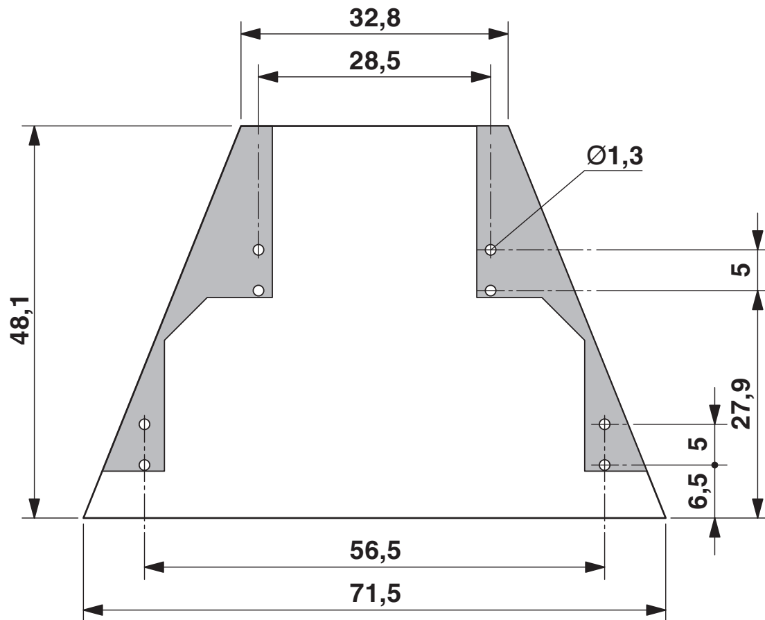
尺寸图
