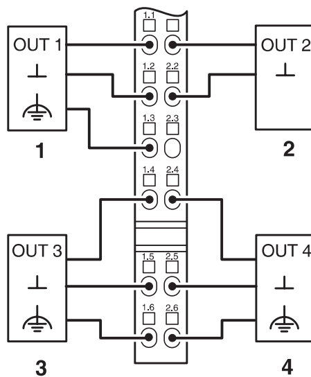
接线图
