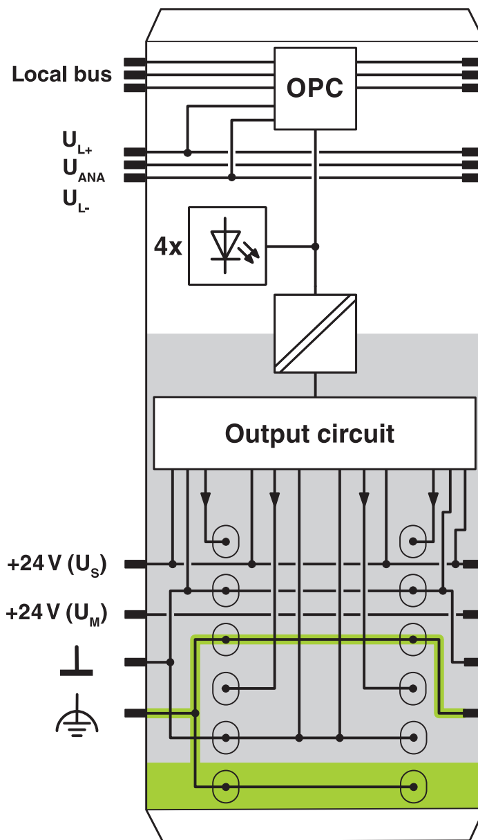
结构框图
