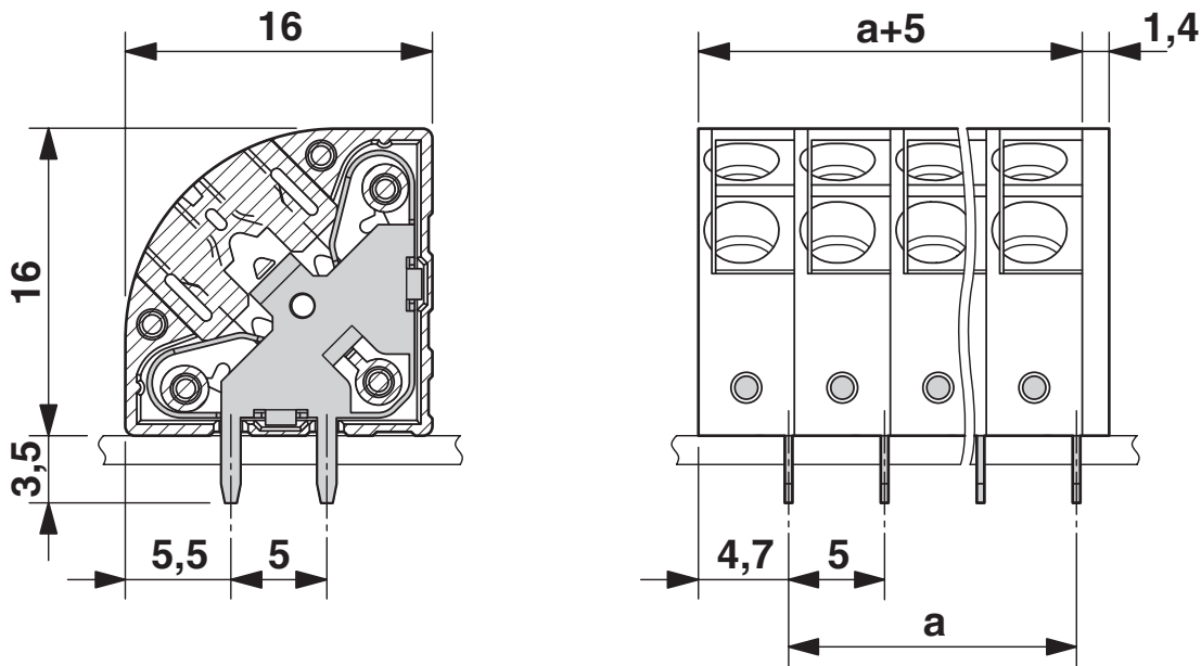
尺寸图
