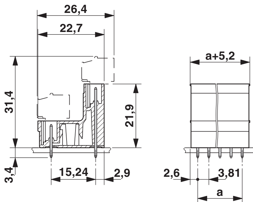
尺寸图
