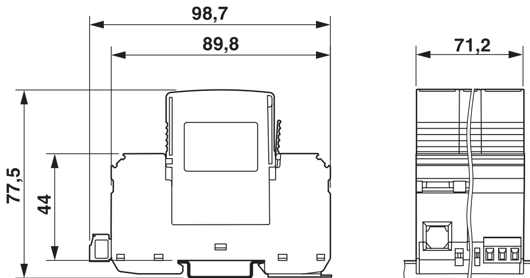
尺寸图
